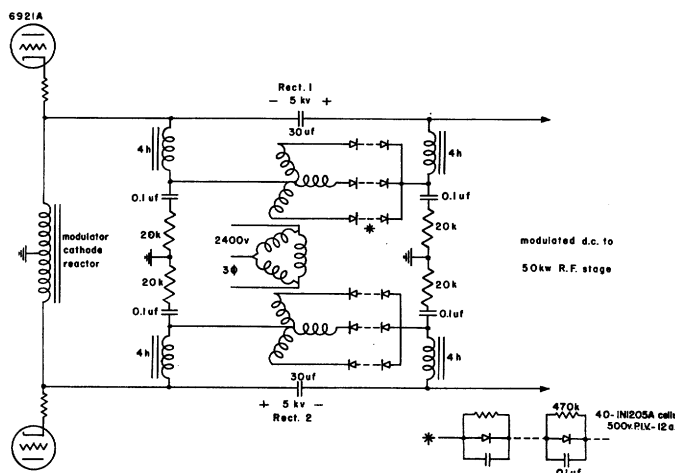
Fig. 16. Split floating rectifiers.
