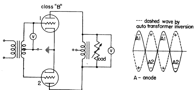
Fig. 7. Anode output W.E. 300B.
