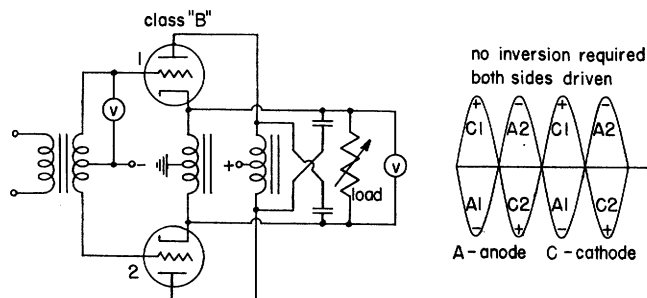
Fig. 9. Cathanode output W.E. 300B.
