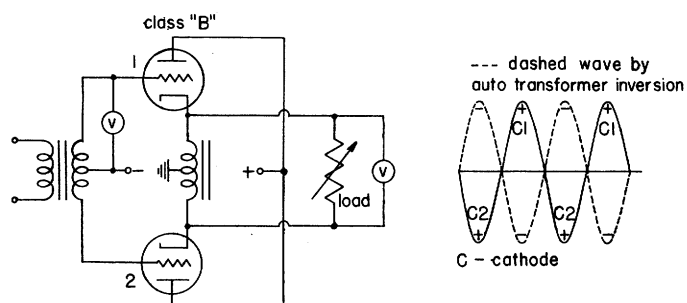
Fig. 8. Cathode output W.E. 300B.
